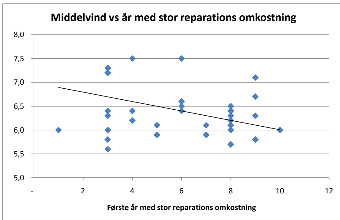
Figur 12 Der ses en trend at jo større middelvindhastighed, des tidligere indtræffer første år med en større reparationsomkostning. Men det er ikke markant entydigt. En "stor" reparationsomkostning er her defineret som > 50 kr/kW.
