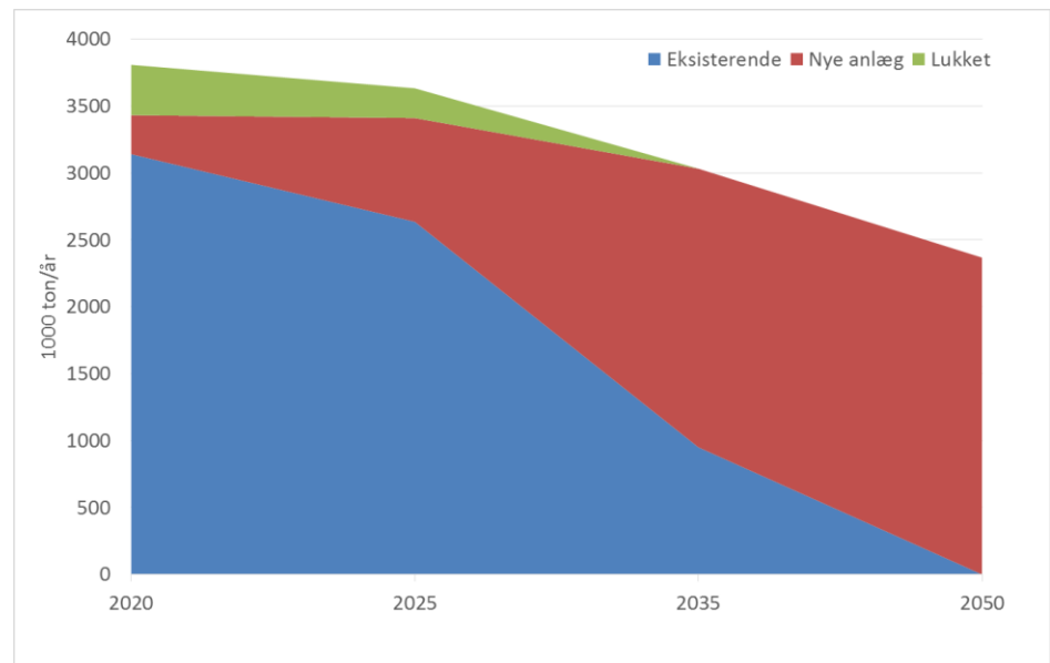
Figur 8. Udvikling af kapacitet i Licitationscenariet for hele Danmark opdelt på eksisterende anlæg (indeholdende planlagte anlæg), nye anlæg og lukkede anlæg. Lukkede anlæg er eksisterende eller planlagte værker, der principielt har ledig ikke-udtjent kapacitet. (1000 tons/år)
