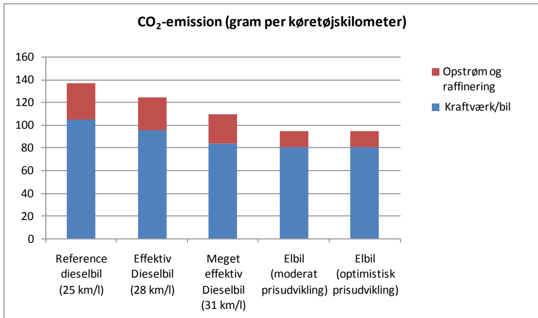
Figur 7: CO 2 -emissioner per køretøjskilometer for hhv. dieselbiler (25 km/l, 28 km/l og 31 km/l) og elbiler i 2020. Tallene ekskluderer opstrømsemmissioner og tab forbundet med raffinering af diesel.
