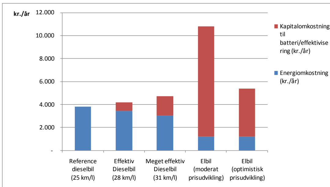
Figur 6: Årlige energikomkostninger, inkl. omkostninger til effektivisering, batteri og ladeinfrastruktur i 2020.
